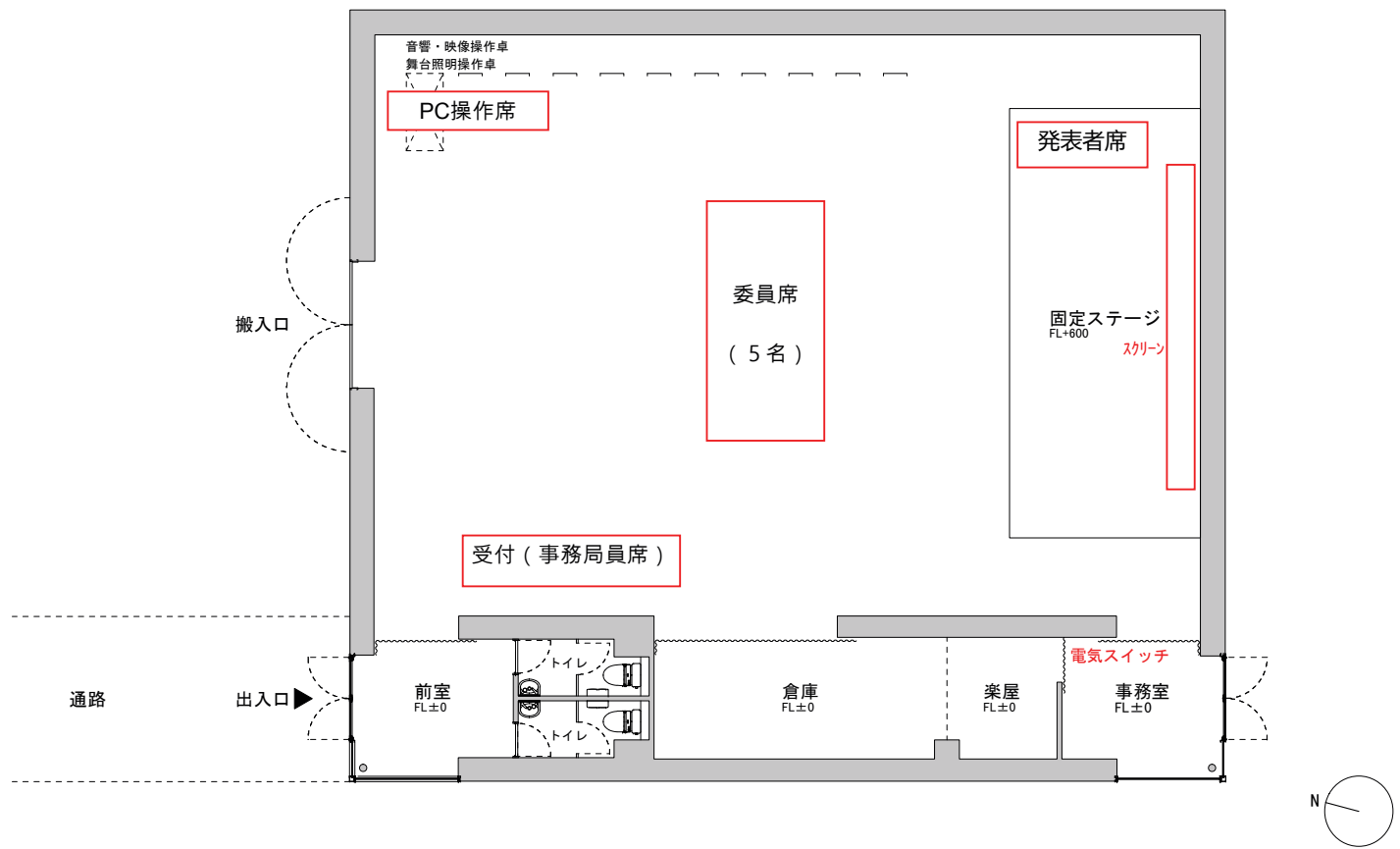
釜石PIT 全体平面図 S=1/100(A3)
