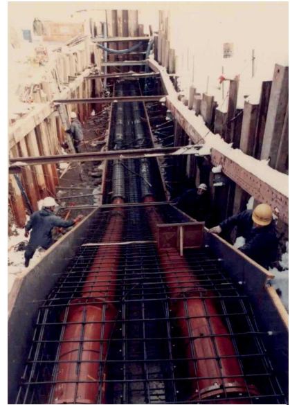
小佐野・中妻污水幹線布設工事 小川川横断の伏せ越し(河川の下を横断)管設置状況。交互に清掃できるように2条化されている
